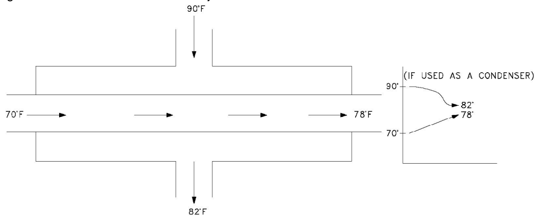
Figure 5: Intercambiador de calor de flujo cruzado.
