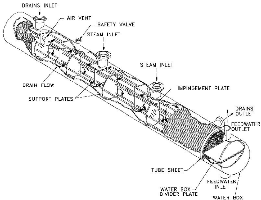
Figure 1: Intercambiador de calor de carcasa y tubos.
