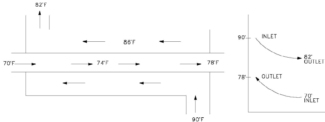
Figure 4: Intercambiador de Contraflujo
