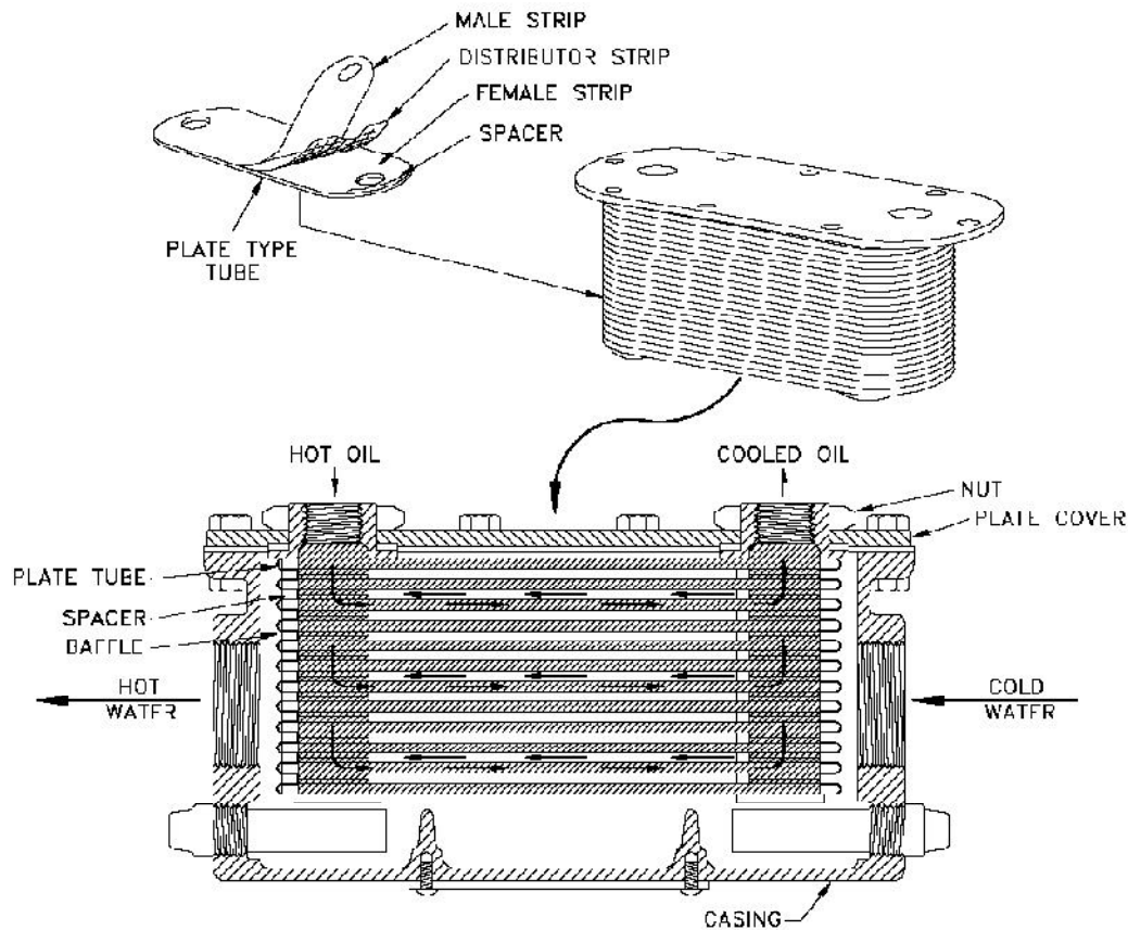
Figure 2: Intercambiador de calor de tipo plato.
