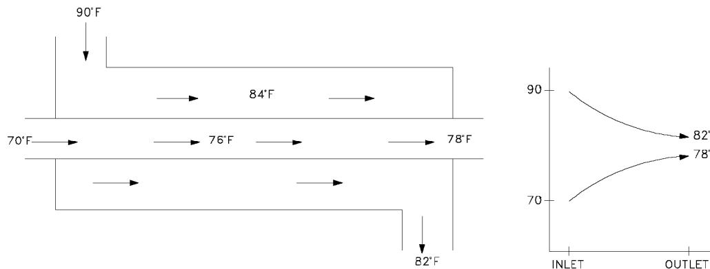
Figure 3: Intercambiador de calor de flujo paralelo.
